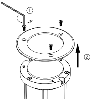
4. 取出安裝筒的蓋子。
